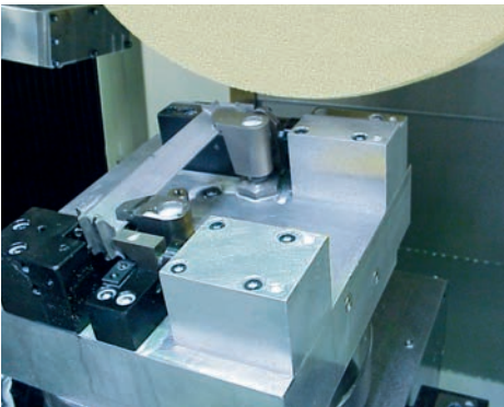
Turbine blade (MC 607)
